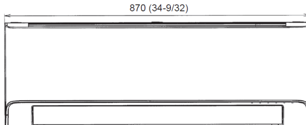
&lt;Front View&gt;
