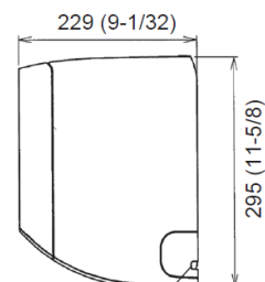
&lt;Side View&gt;
